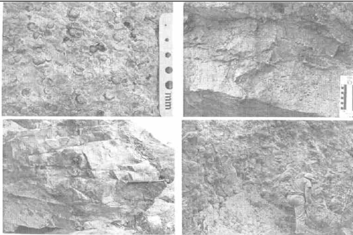
图1 火山岩亚相图片
