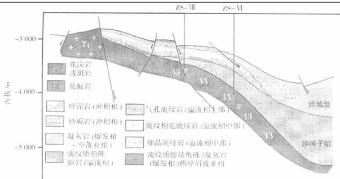
图3 松辽盆地 VII 0 线构造剖面 ZS-VIII 井-ZS-VI 井火山岩岩相对比与储层预测剖面
