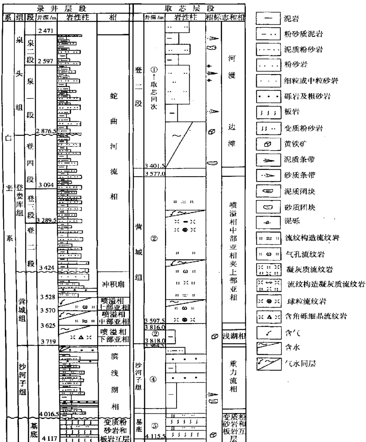
图2 ZS-VI井深层火山岩-沉积岩岩相分析
